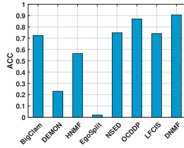
Fig. 3: Node-level analysis.
